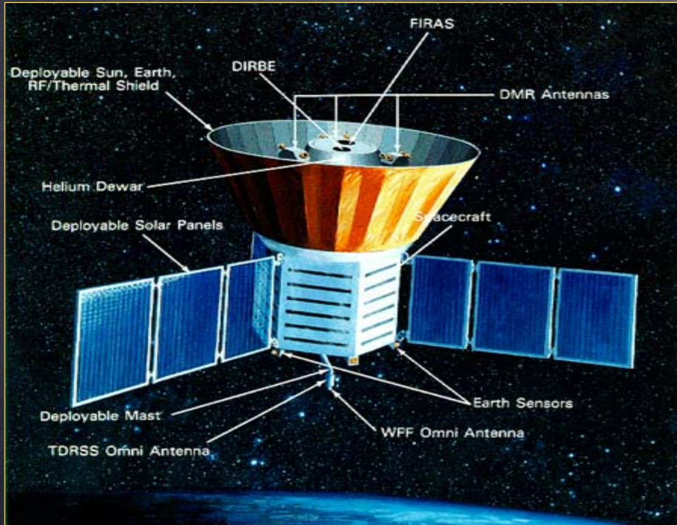
COBE (1989 - 1994)
